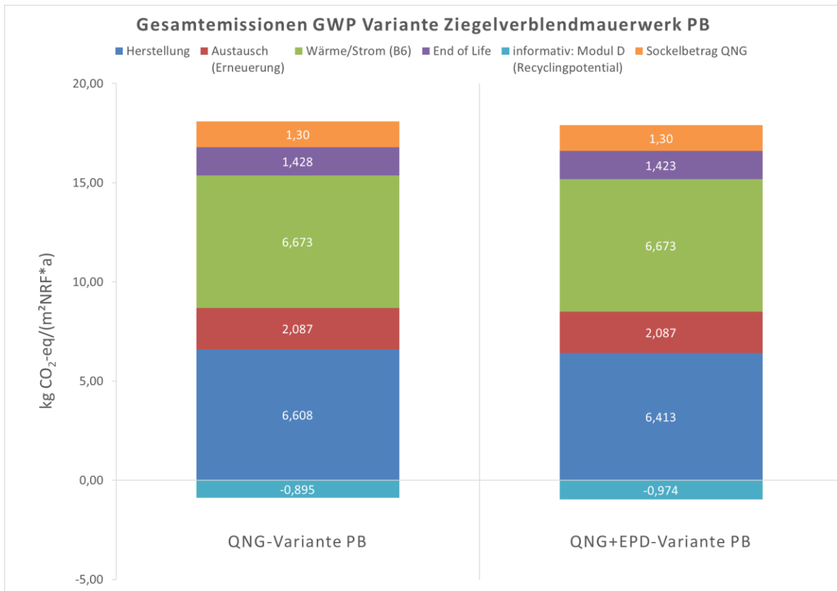
Abb. 4-1: Gesamtergebnisse Variante Ziegelverblendmauerwerk PB für CO 2 -Äquivalente
