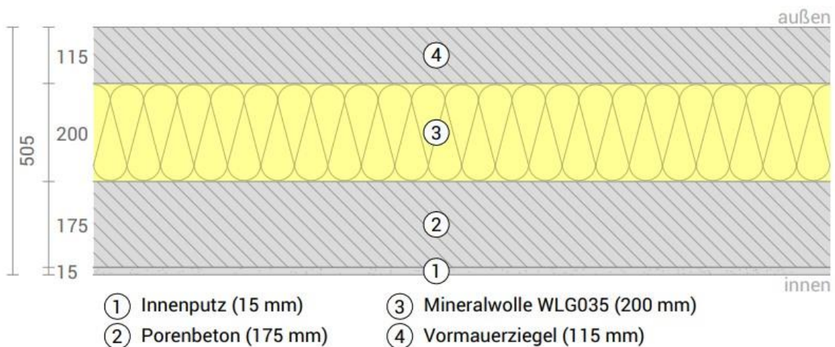
Abb. 3-2: Konfiguration Außenwand Porenbeton-Variante
