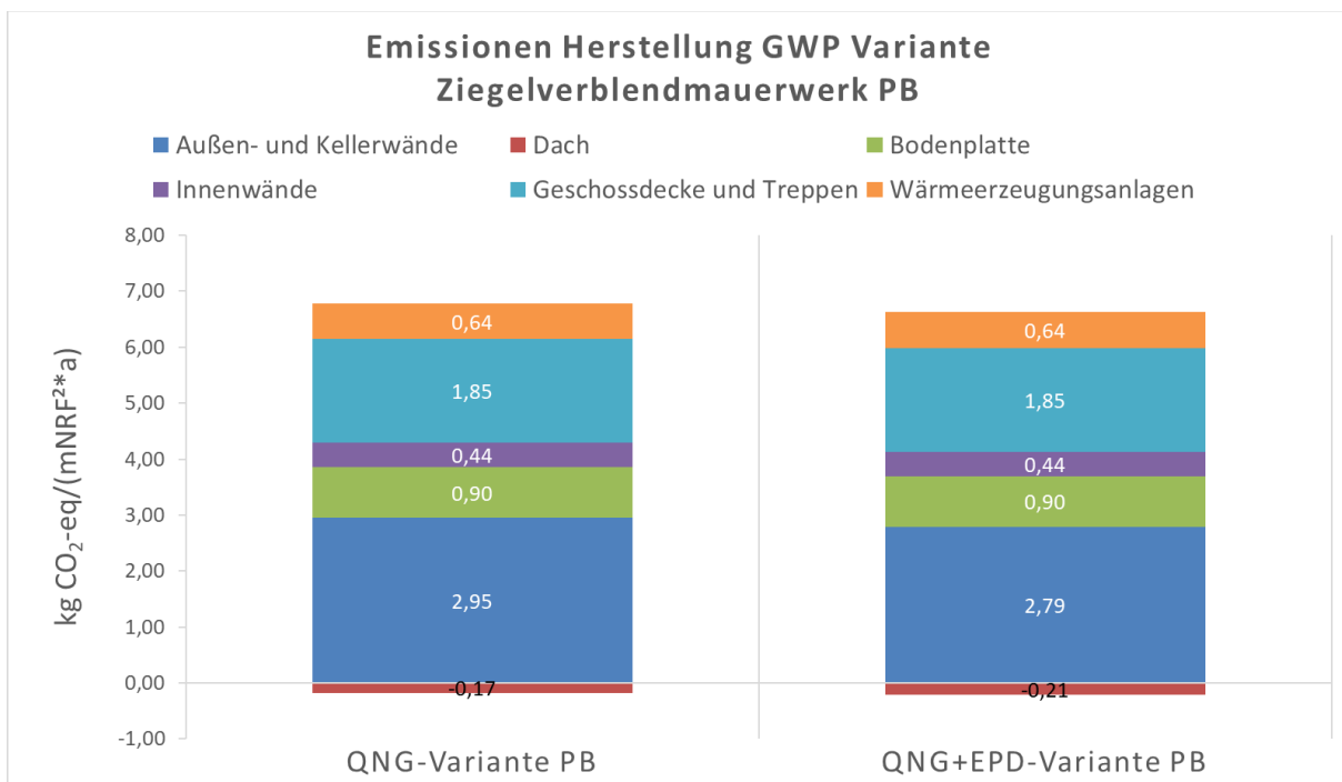
Abb. 4-2: Ergebnisse Herstellungsphase Variante Ziegelverblendmauerwerk PB für CO 2 -Äquivalente
