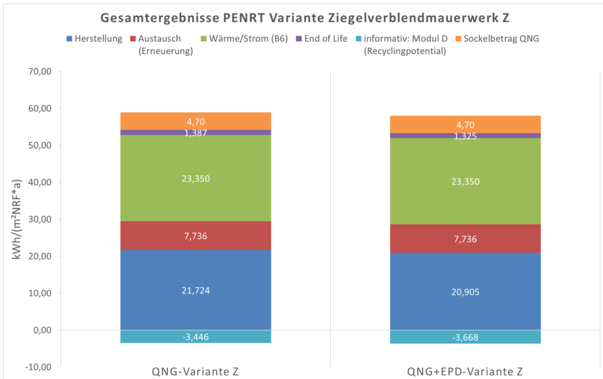
Abb. 4-7: Gesamtergebnisse Variante Ziegelverblendmauerwerk Z für PE nicht erneuerbar
