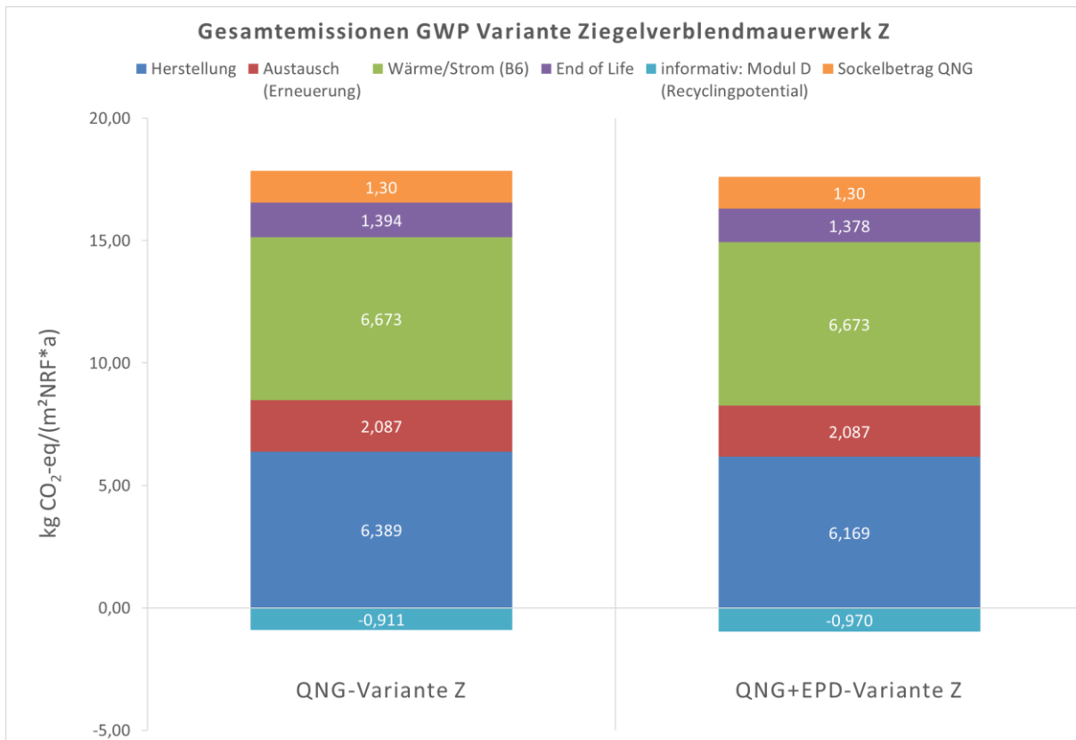
Abb. 4-5: Gesamtergebnisse Variante Ziegelverblendmauerwerk Z für CO 2 -Äquivalente
