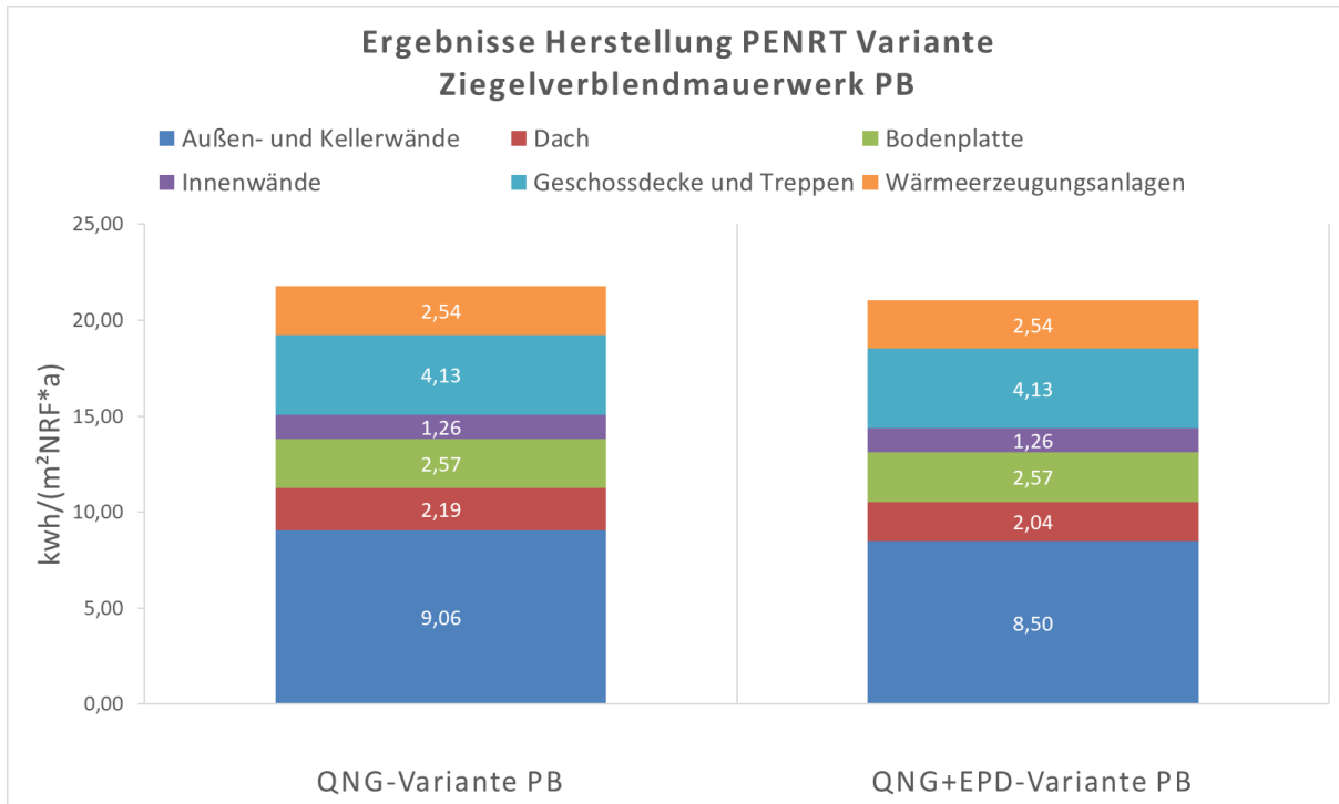
Abb. 4-4: Ergebnisse Herstellungsphase Variante Ziegelverblendmauerwerk PB für PE nicht erneuerbar
