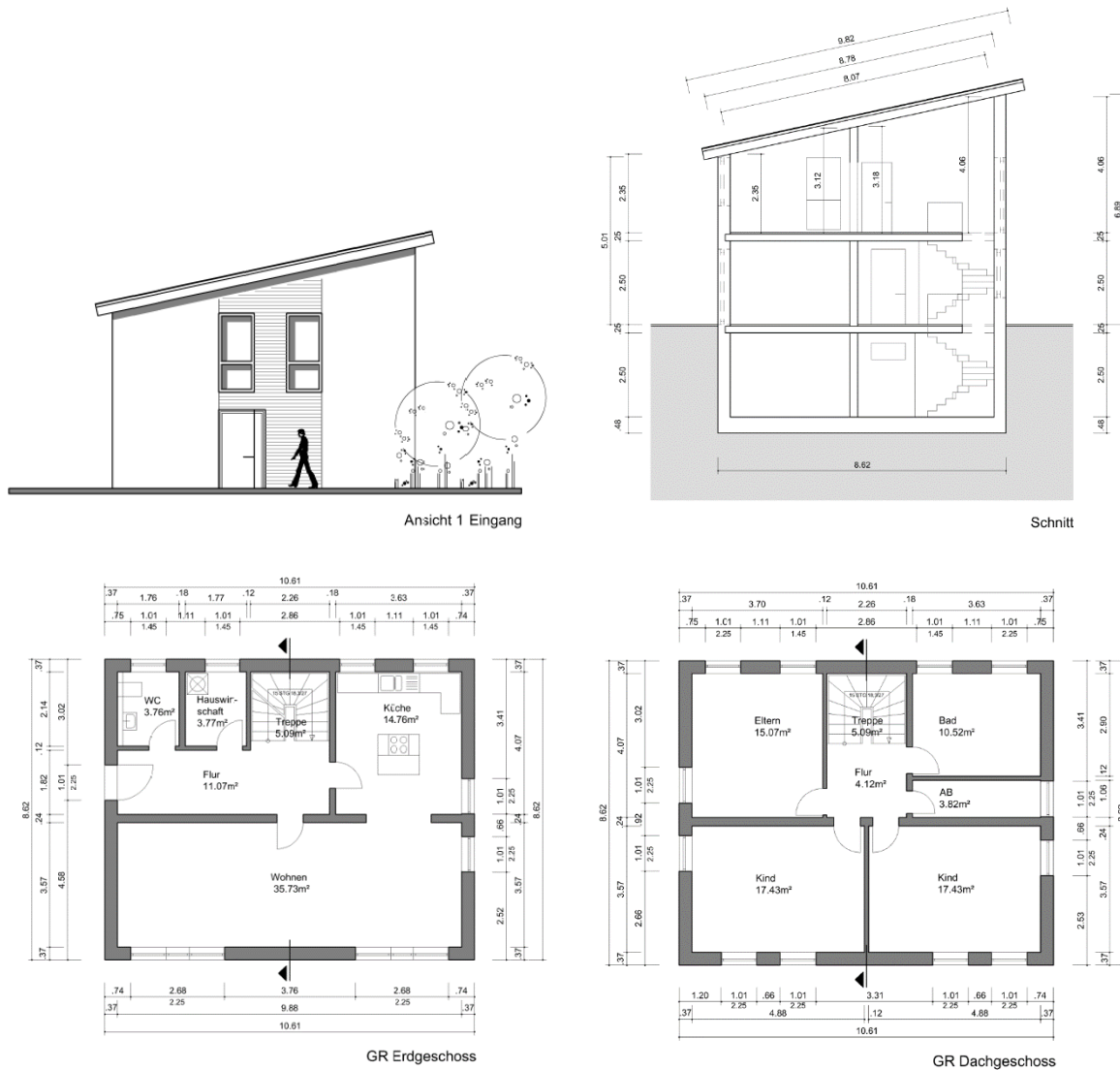
Abb. 3-1: Ansicht, Schnitt, Grundrisse und Daten zu Muster-EFH (Quelle: Arge Kiel e.V)
