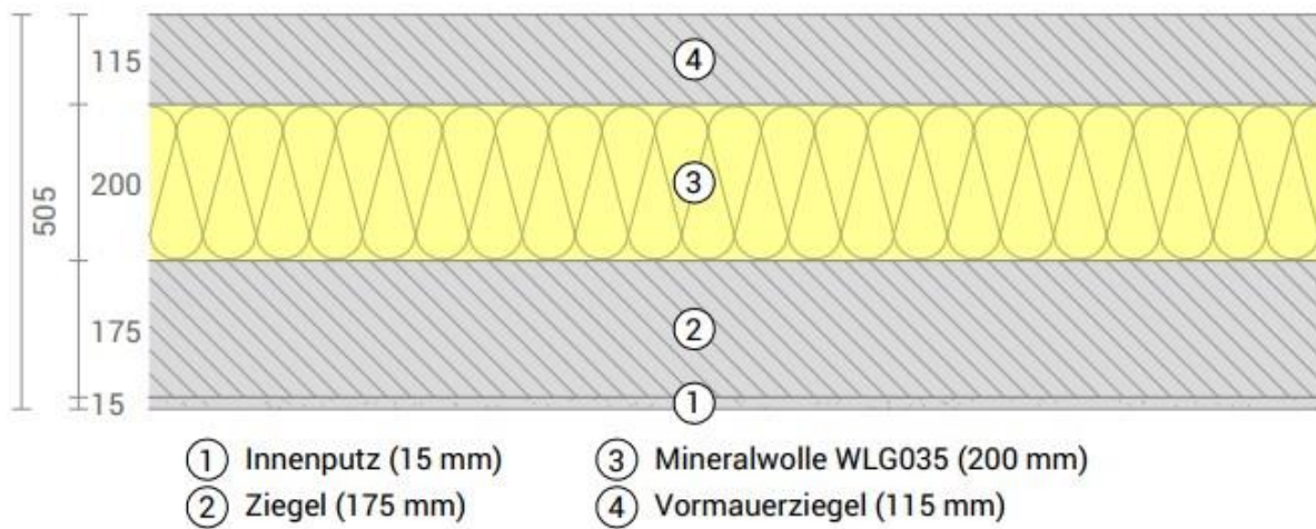
Abb. 3-3: Konfiguration Außenwand Ziegel (ungefüllt)-Variante
