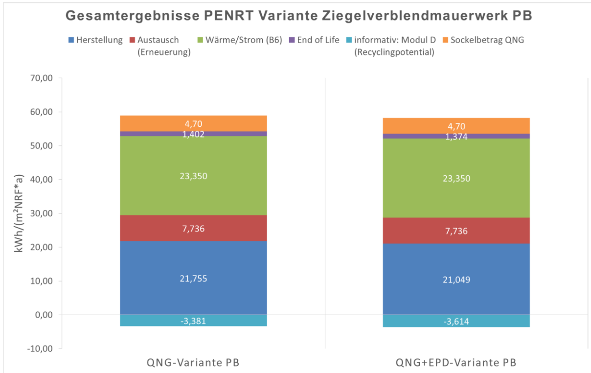
Abb. 4-3: Gesamtergebnisse Variante Ziegelverblendmauerwerk PB für PE nicht erneuerbar
