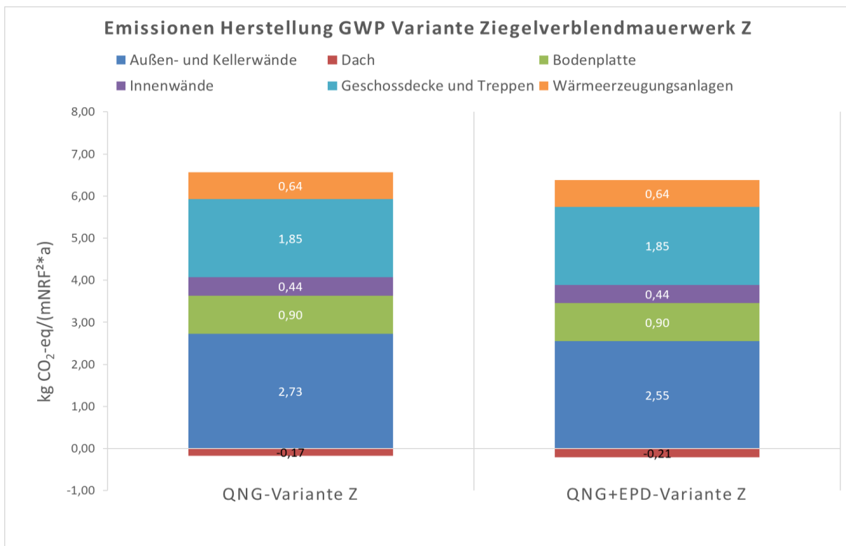
Abb. 4-6: Ergebnisse Herstellungsphase Variante Ziegelverblendmauerwerk Z für CO 2 -Äquivalente
