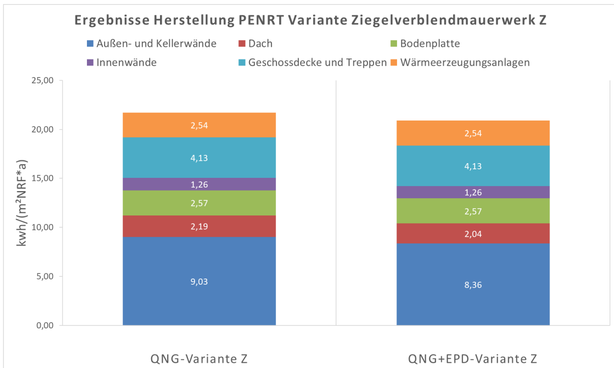
Abb. 4-8: Ergebnisse Herstellungsphase Variante Ziegelverblendmauerwerk Z für PE nicht erneuerbar
